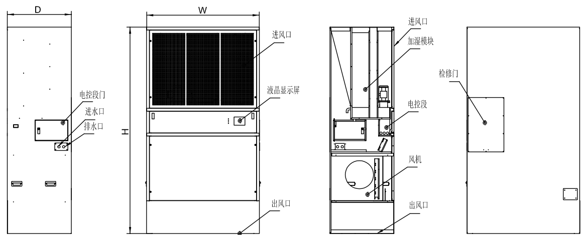
Condair PH系列下送风外观图
