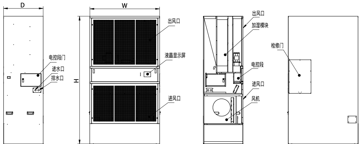
Condair PH系列上送风外观图
